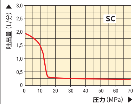
吐出量曲線
